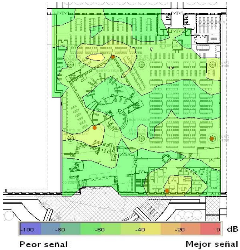
Mapa cobertura Biblioteca Planta Baja Red Oviwan
