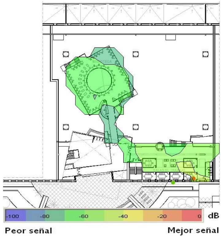
Mapa Cobertura Biblioteca Primera Planta Red Wupolan
