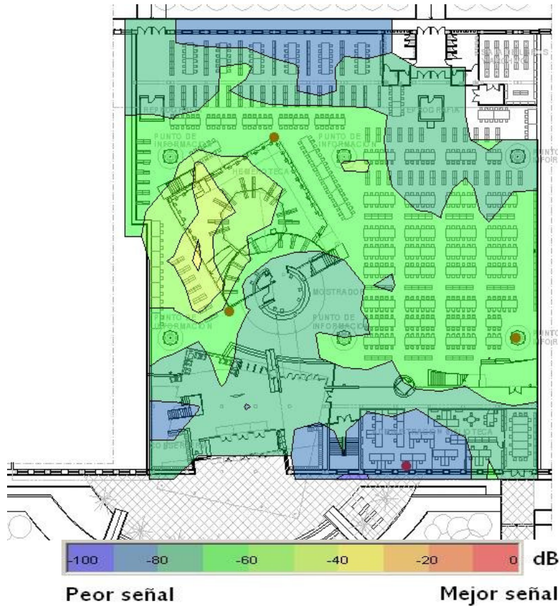
Mapa Cobertura Biblioteca Planta Baja Red Wupolan
