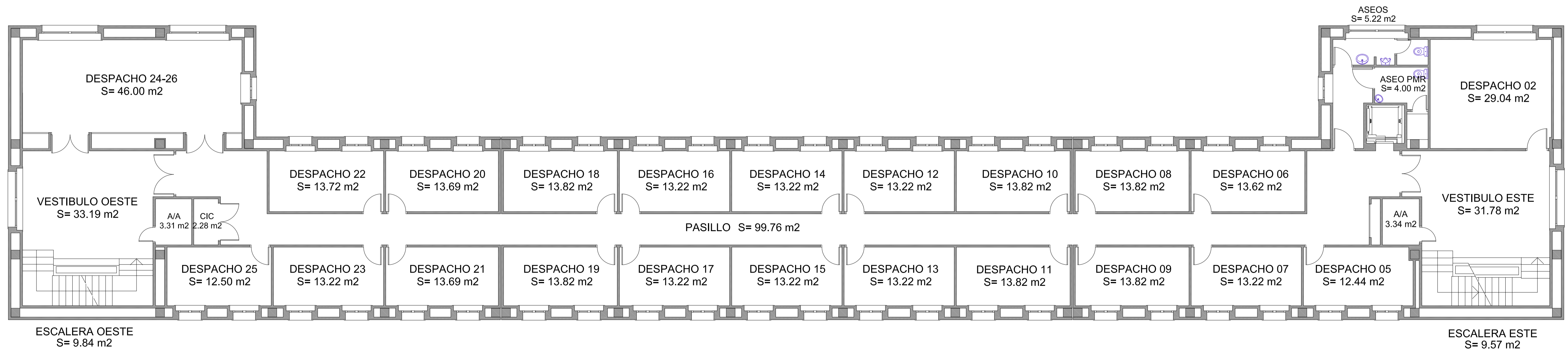
PLANTA SEGUNDA
