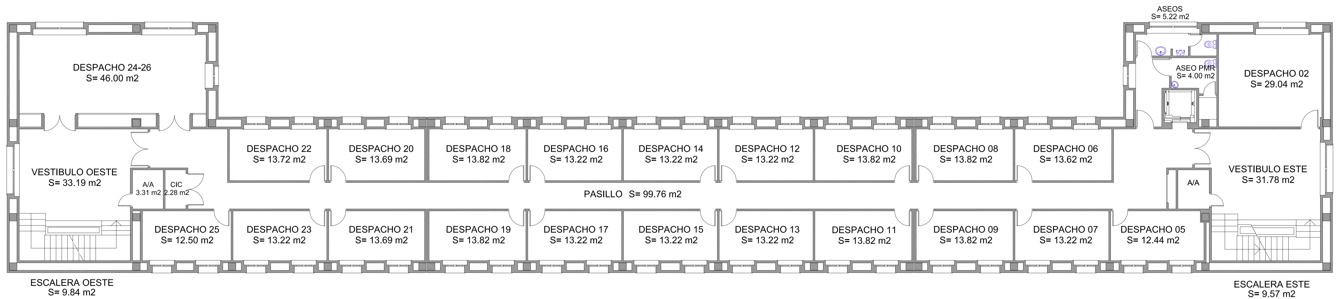
PLANTA TERCERA
