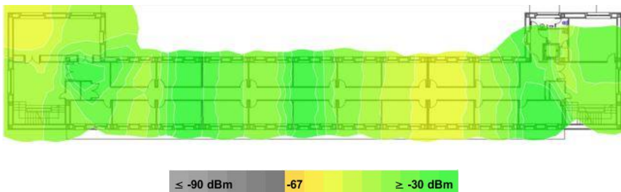
Grafico 4: Cobertura eduroam y wupolan Edificio 11 planta 3.
