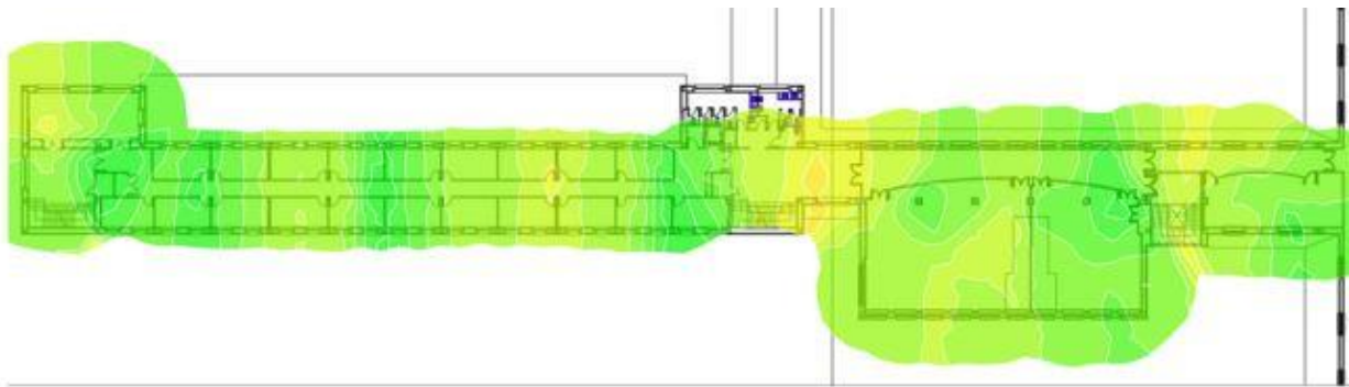
Grafico 1: Cobertura eduroam y wupolan Edificio 11 planta baja.
