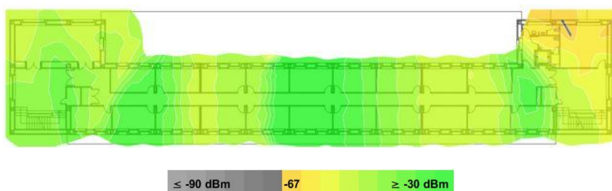
Grafico 5: Cobertura eduroam y wupolan Edificio 11 planta 4.
