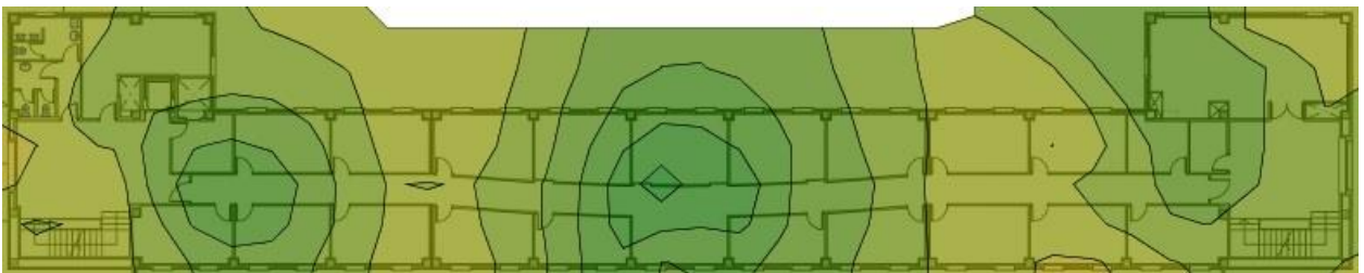
Grafico 5: Cobertura eduroam Edificio 2 planta 4.
