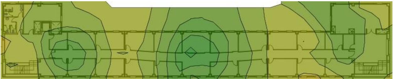
Grafico 6: Cobertura wupolan Edificio 2 planta 3.
