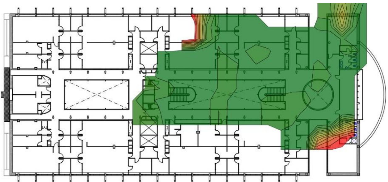
Grafico 5: Cobertura eduroam Edificio 20 planta 2.
