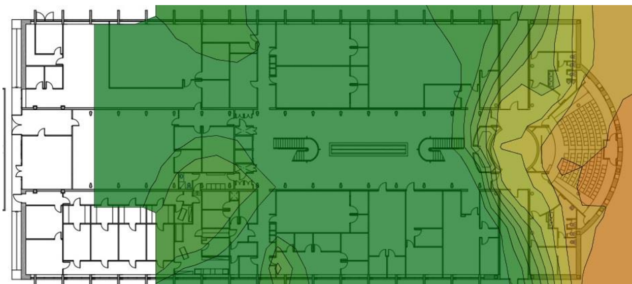
Grafico 1: Cobertura eduroam Edificio 20 planta baja.
