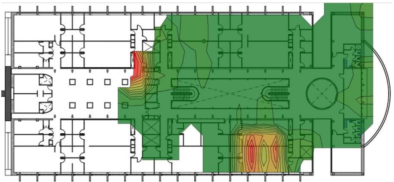
Grafico 3: Cobertura eduroam Edificio 20 planta 1.
