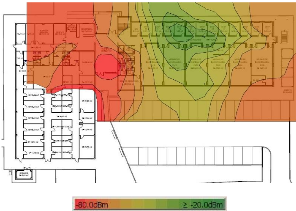
Grafico 1: Cobertura eduoram Edificio 21 planta baja.
