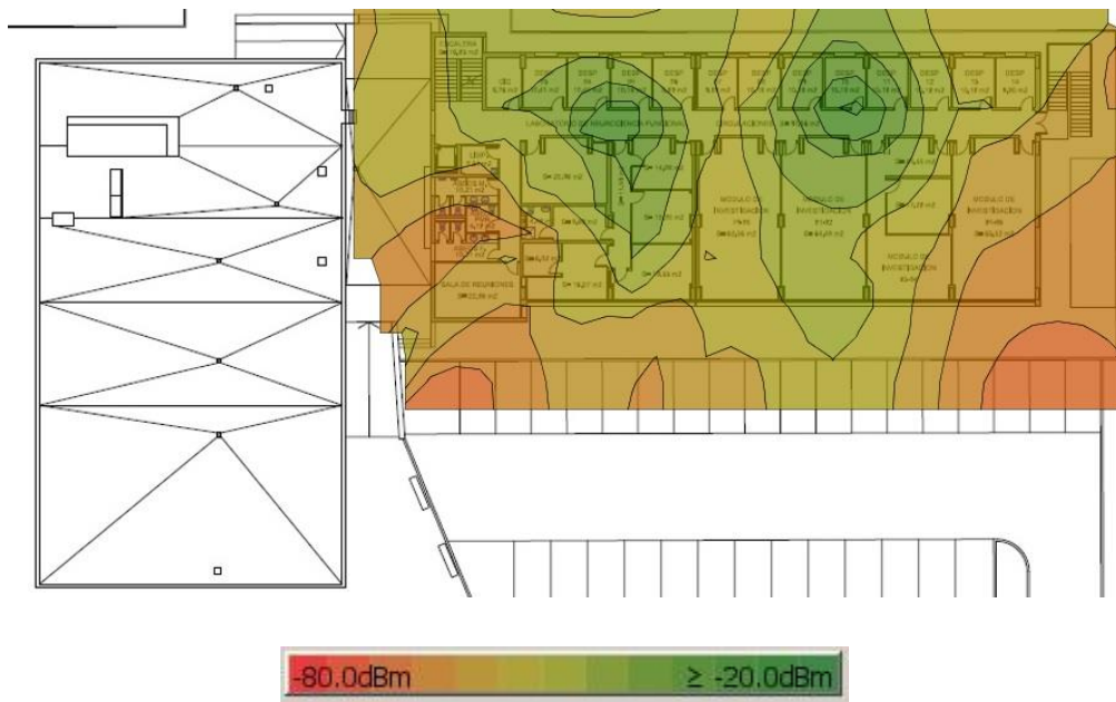
Grafico 4: Cobertura wupolan Edificio 21 planta 1.
