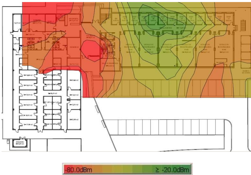
Grafico 2: Cobertura wupolan Edificio 21 planta baja.
