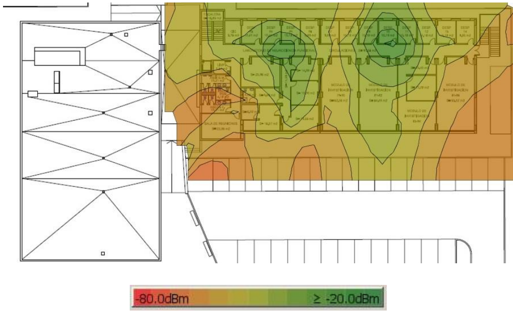
Grafico 3: Cobertura eduroam Edificio 21 planta 1.
