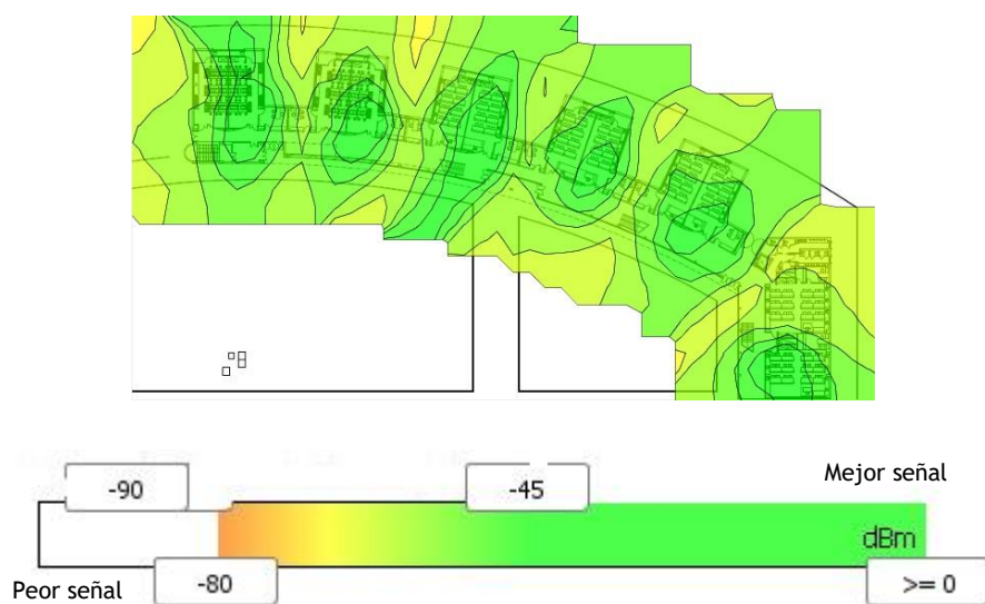
Grafico 2: Cobertura wupolan Edificio 23 planta baja.
