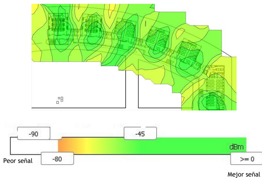
Grafico 1: Cobertura eduroam Edificio 23 planta baja.
