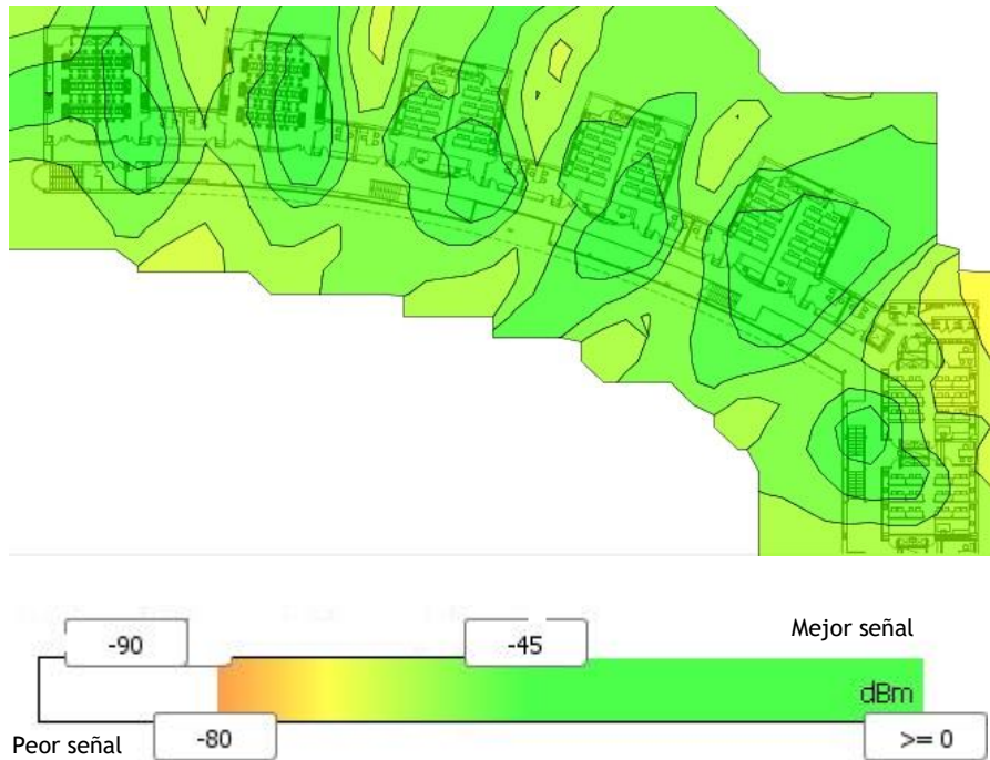
Grafico 3: Cobertura eduroam Edificio 23 planta 2.
