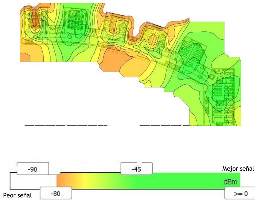
Grafico 4: Cobertura wupolan Edificio 23 planta 1.
