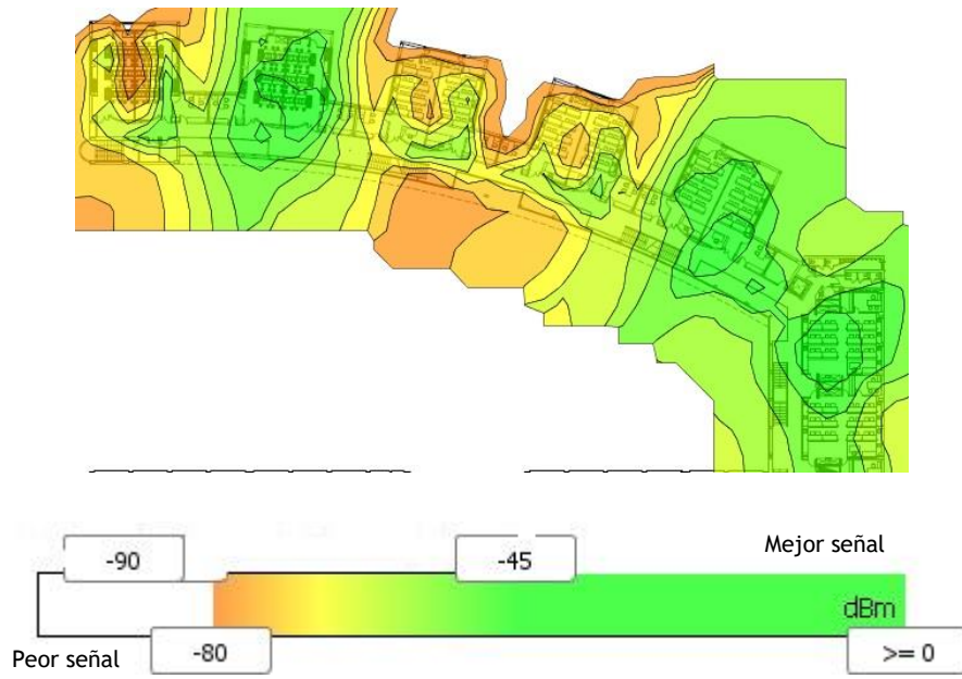
Grafico 3: Cobertura eduroam Edificio 23 planta 1.
