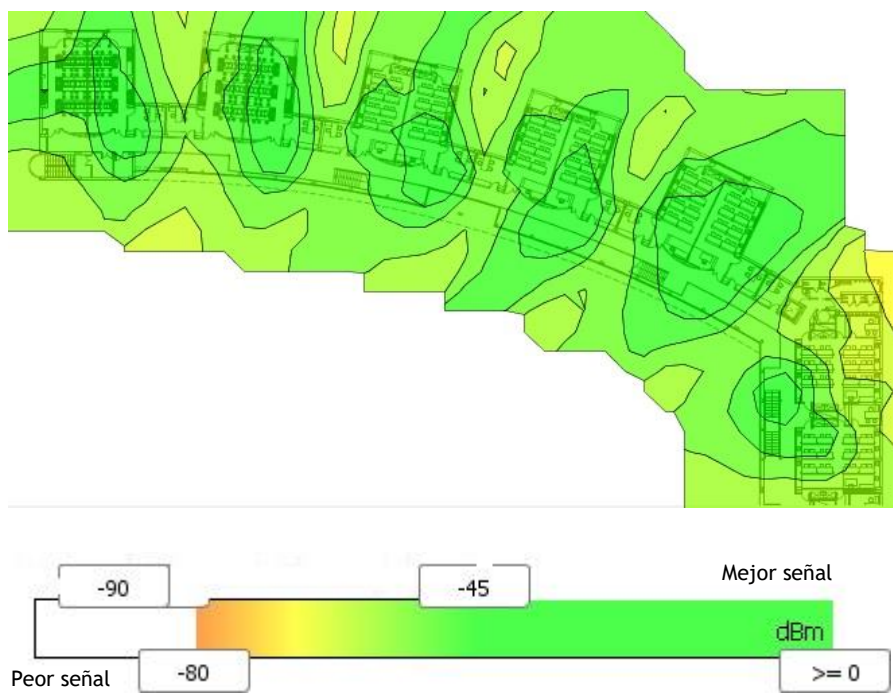
Grafico 3: Cobertura eduroam Edificio 23 planta 2.
