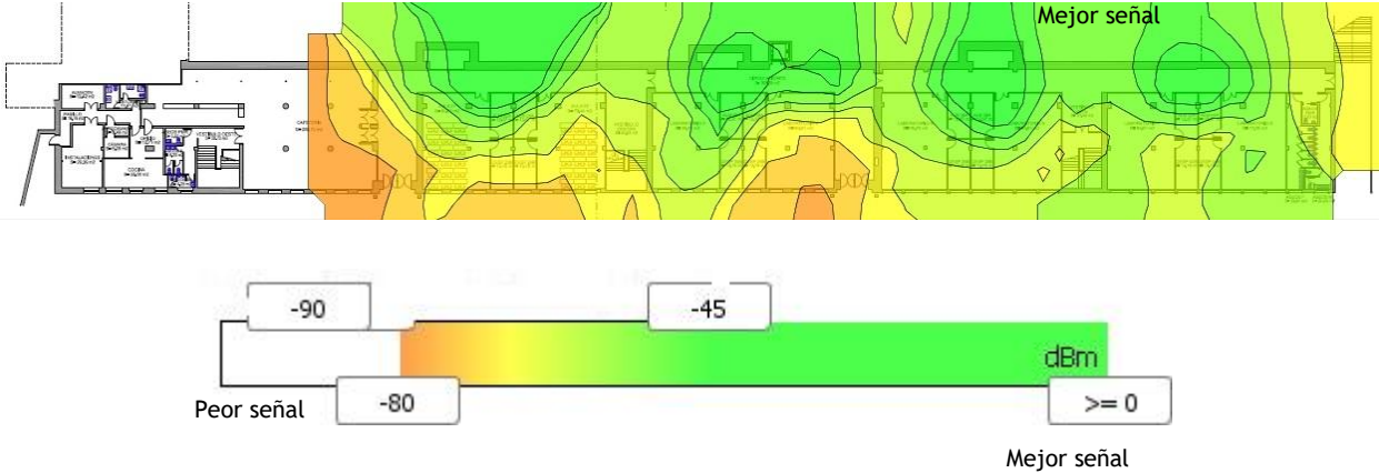
Grafico 2: Cobertura wupolan Edificio 24-29 planta sótano.
