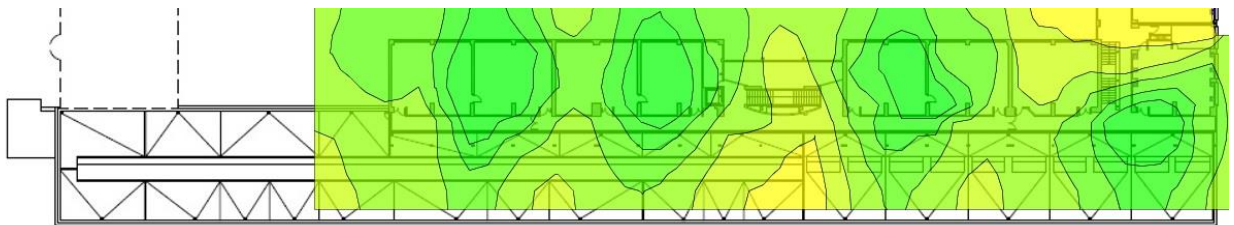
Grafico 5: Cobertura eduroam Edificio 24-29 planta 2.
