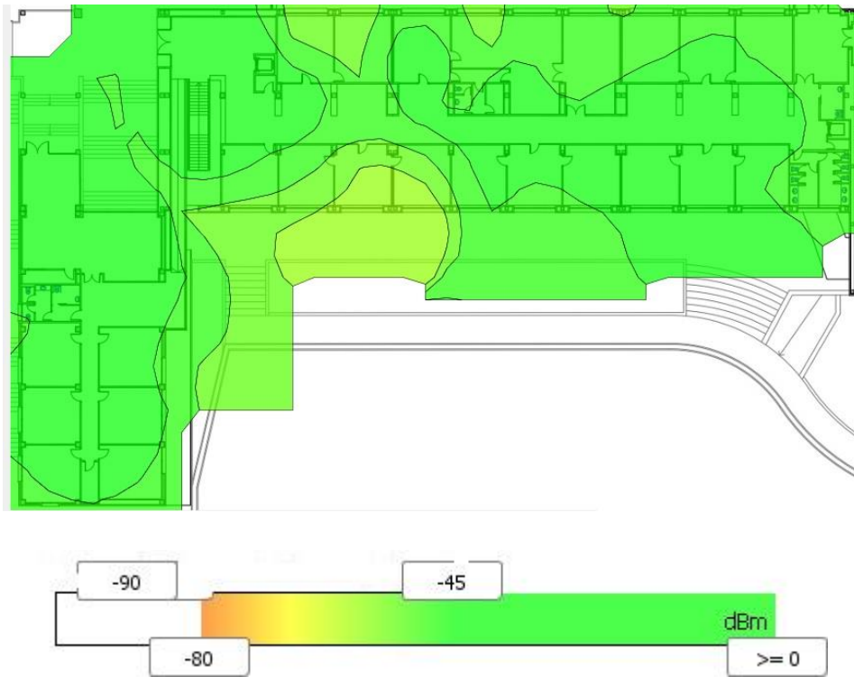
Grafico 4: Cobertura wupolan Edificio 32 planta 1.
