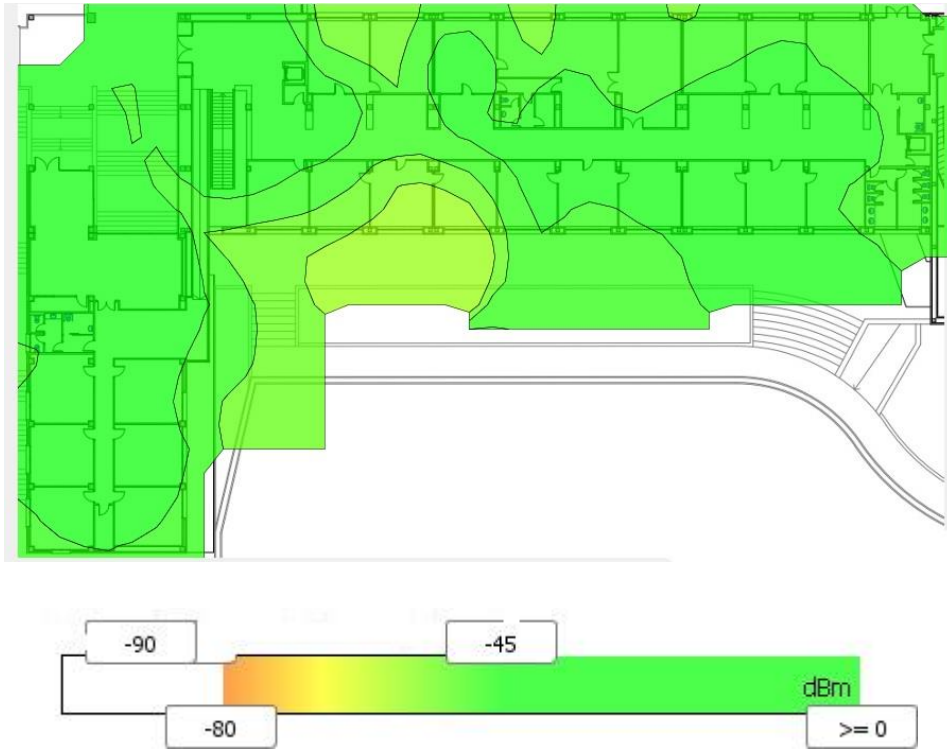
Grafico 3: Cobertura eduroam Edificio 32 planta 1.
