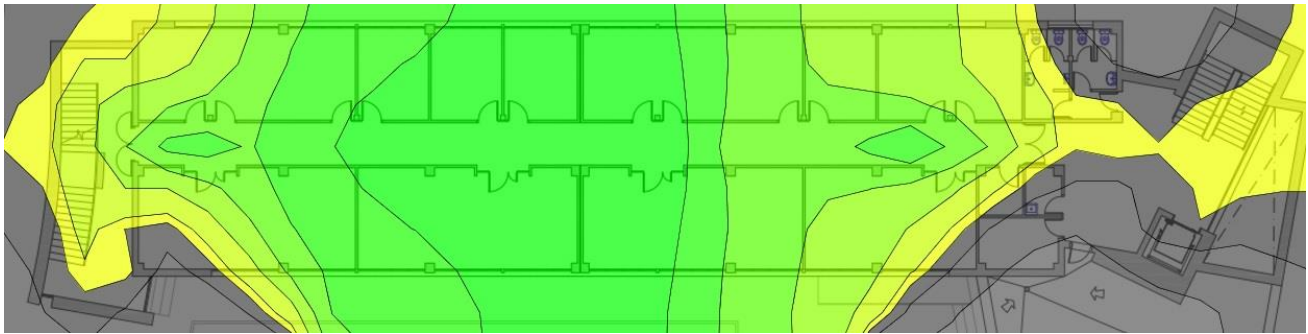
Grafico 3: Cobertura eduroam Edificio 44 planta 1.
