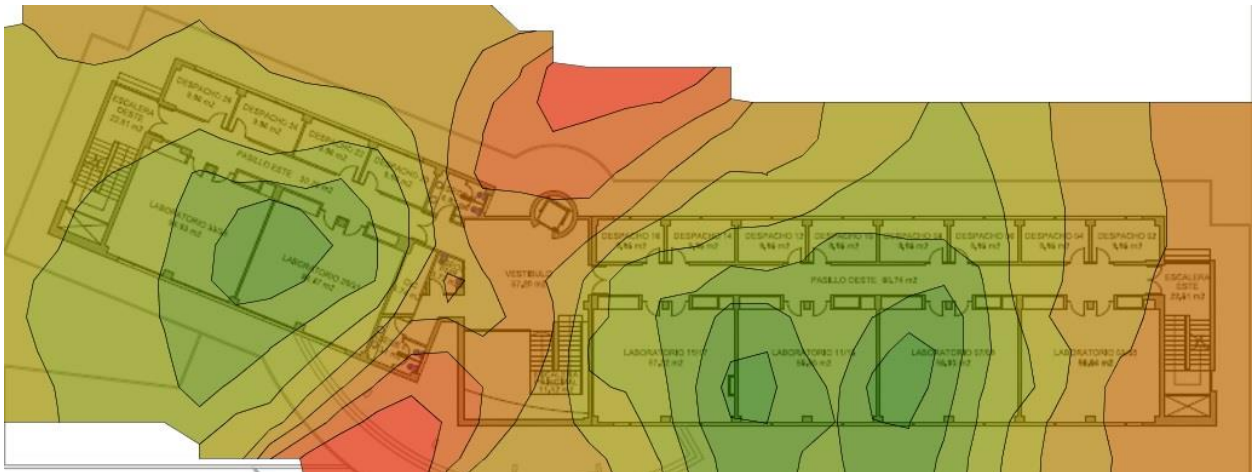
Grafico 3: Cobertura eduroam Edificio 47 planta 1.
