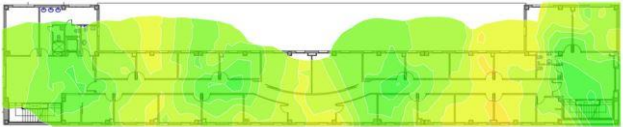
Grafico 4: Cobertura eduroam y wupolan Edificio 6 planta 3.
