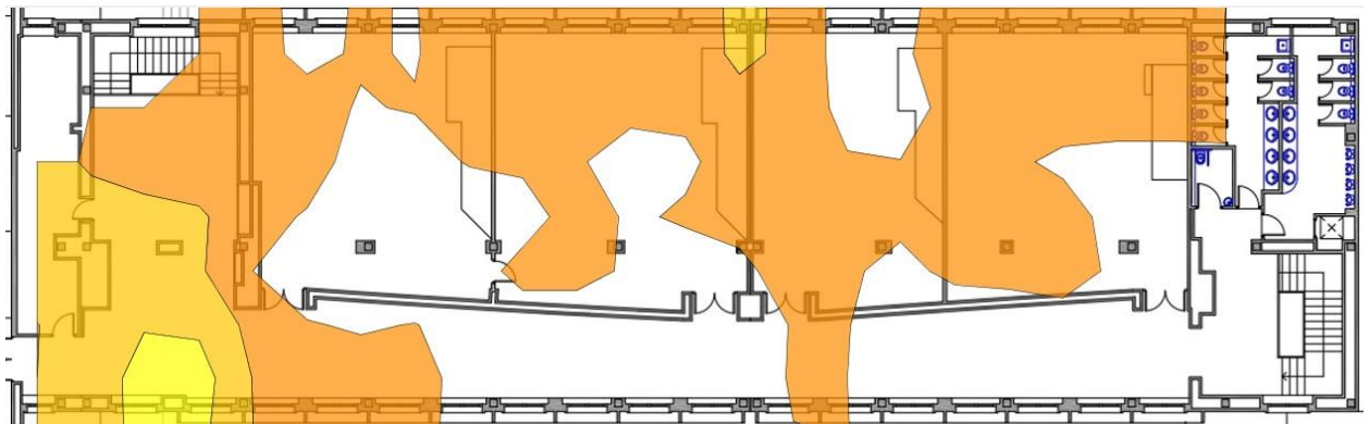
Grafico 3: Cobertura eduroam Edificio 8 planta 1.
