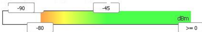
Grafico 3: Cobertura eduroam Galería planta 1.
