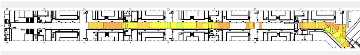
Grafico 1: Cobertura eduroam Galería planta baja.
