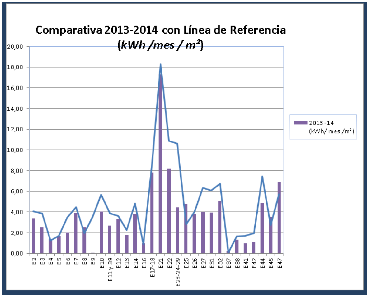
Comparativa 2013-2014 con Línea de Referencia (kWh / mes / m 2 )
