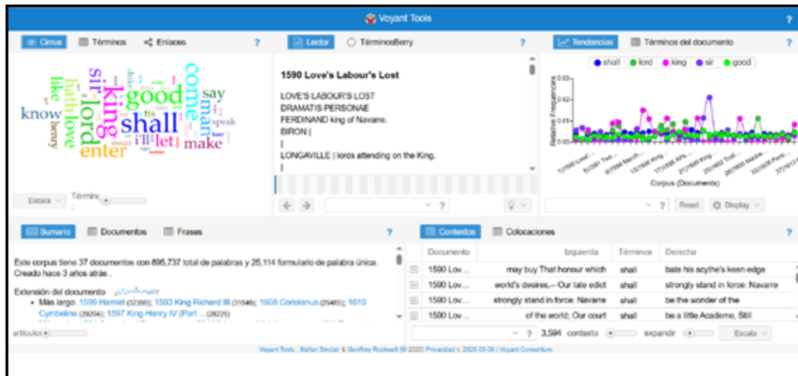
Figura 1. Interfaz de Voyant Tools con un corpus de obras de Shakespeare precargado y sus cinco funciones principales
