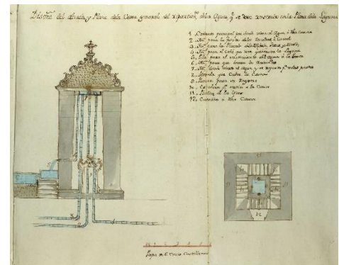
Plano de caja de aguas
