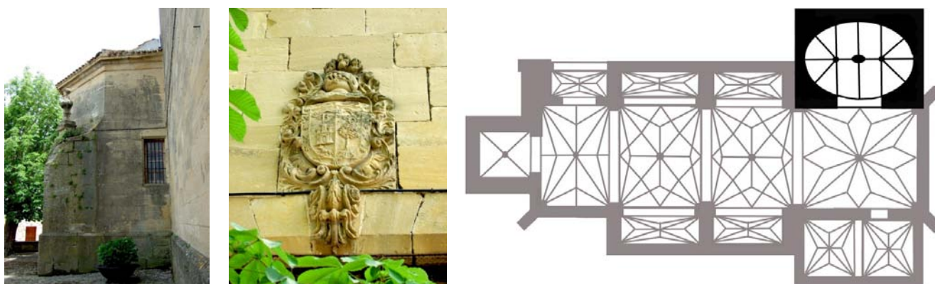
Fig. 2. Planta original y detalle del alzado exterior de Capilla de la Virgen de Guadalupe en la iglesia parroquial de Castañares de Rioja, levantada a expensas de Manuel Silvestre Pérez de Camino entre 1753 y 1757.
